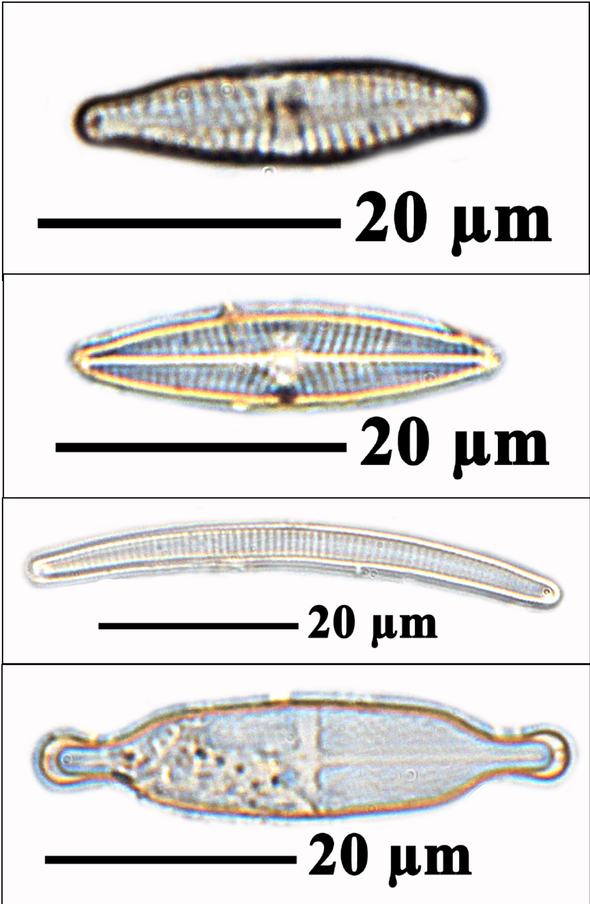
Diatomen aus dem Hölzersee bei Stuttgart, Naphrax
