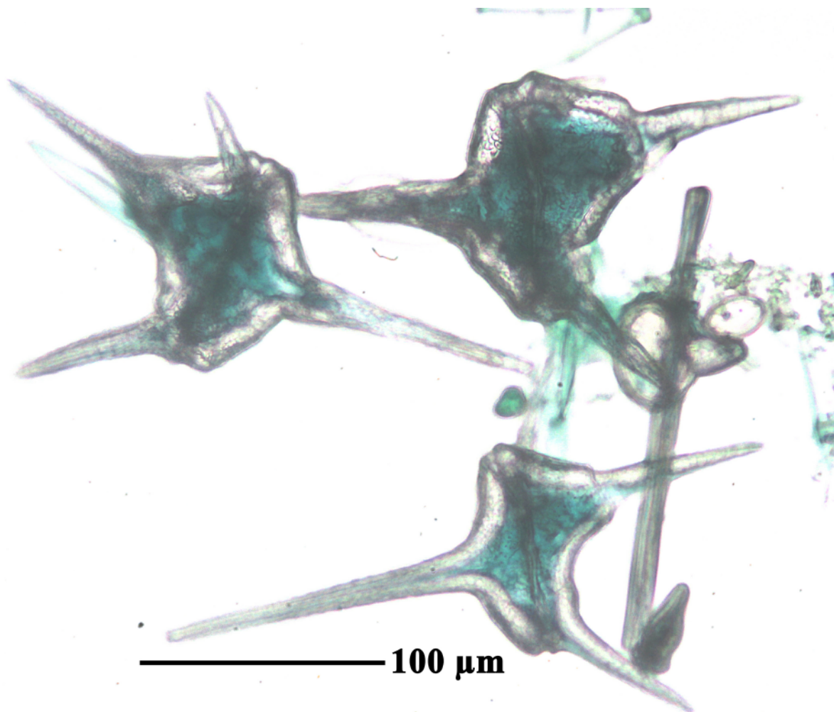
Ceratium hirundinella vom Bärensee bei Stuttgart, Pfeiffer, Alizarinviridin, Glycerin-Gelatine
