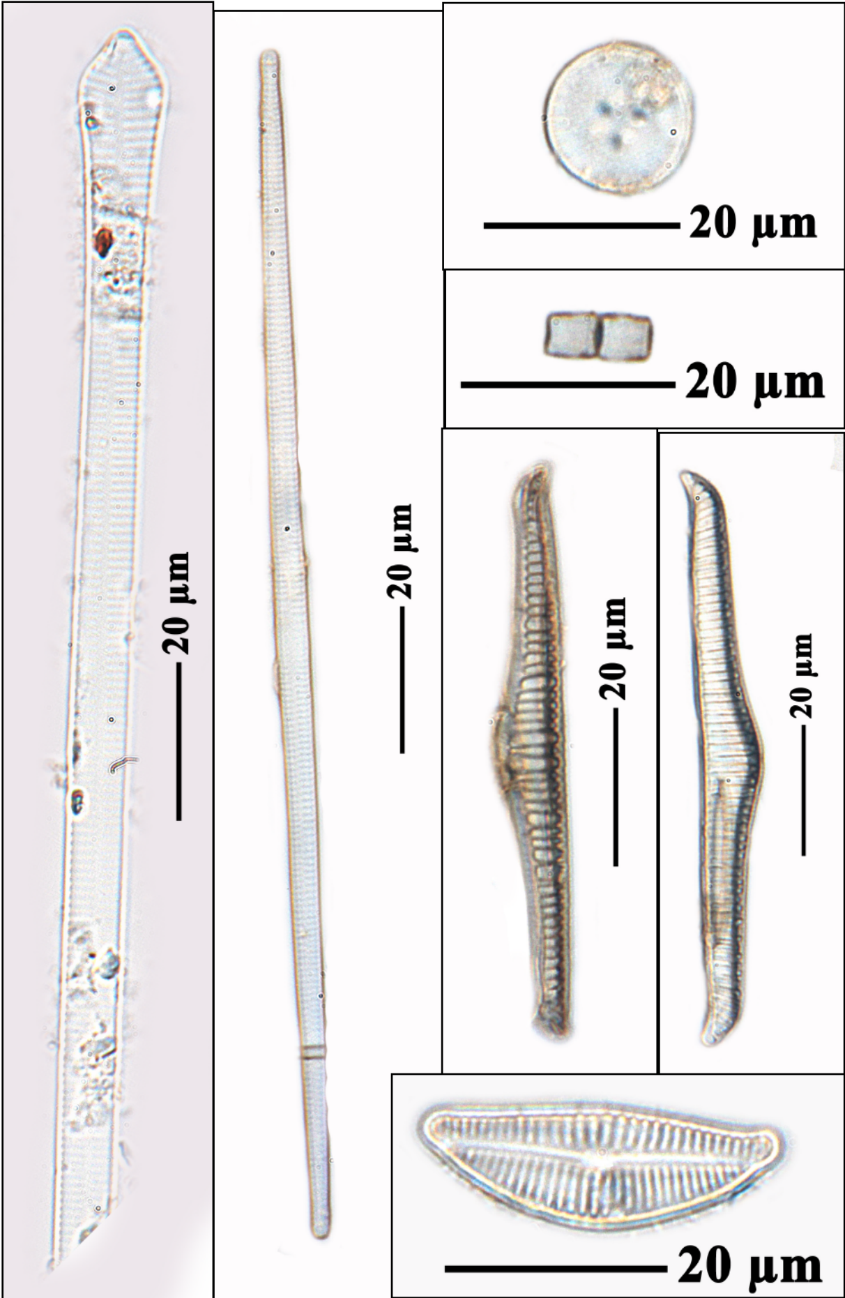
Diatomeen aus dem Pfaffensee bei Stuttgart, Naphrax
