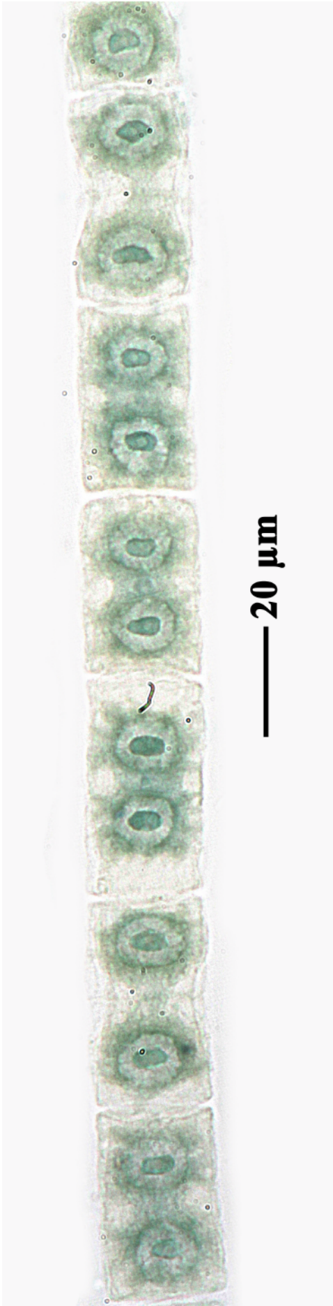
Zygnema leiospermum, Alizarinviridin, Glycerin-Gelatine 2. Bild mit Zygoten
