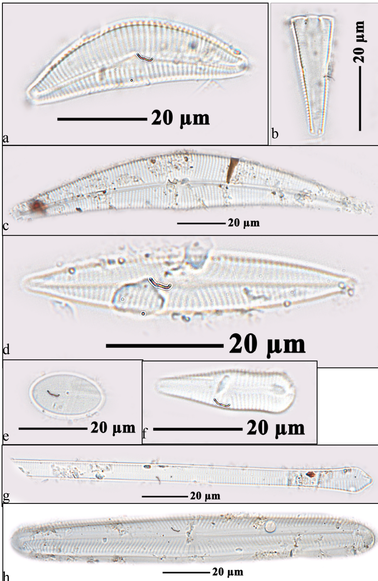
Diatomeen aus dem Bodensee, a: Cymbella ventricosa , b: Rholcosphenia , c: Cymbella lanceolata , d: Navicula radiosa e: Cocconeis lplacentula , f: Gomphonema constrictum , g: Synedra capitata , h:
